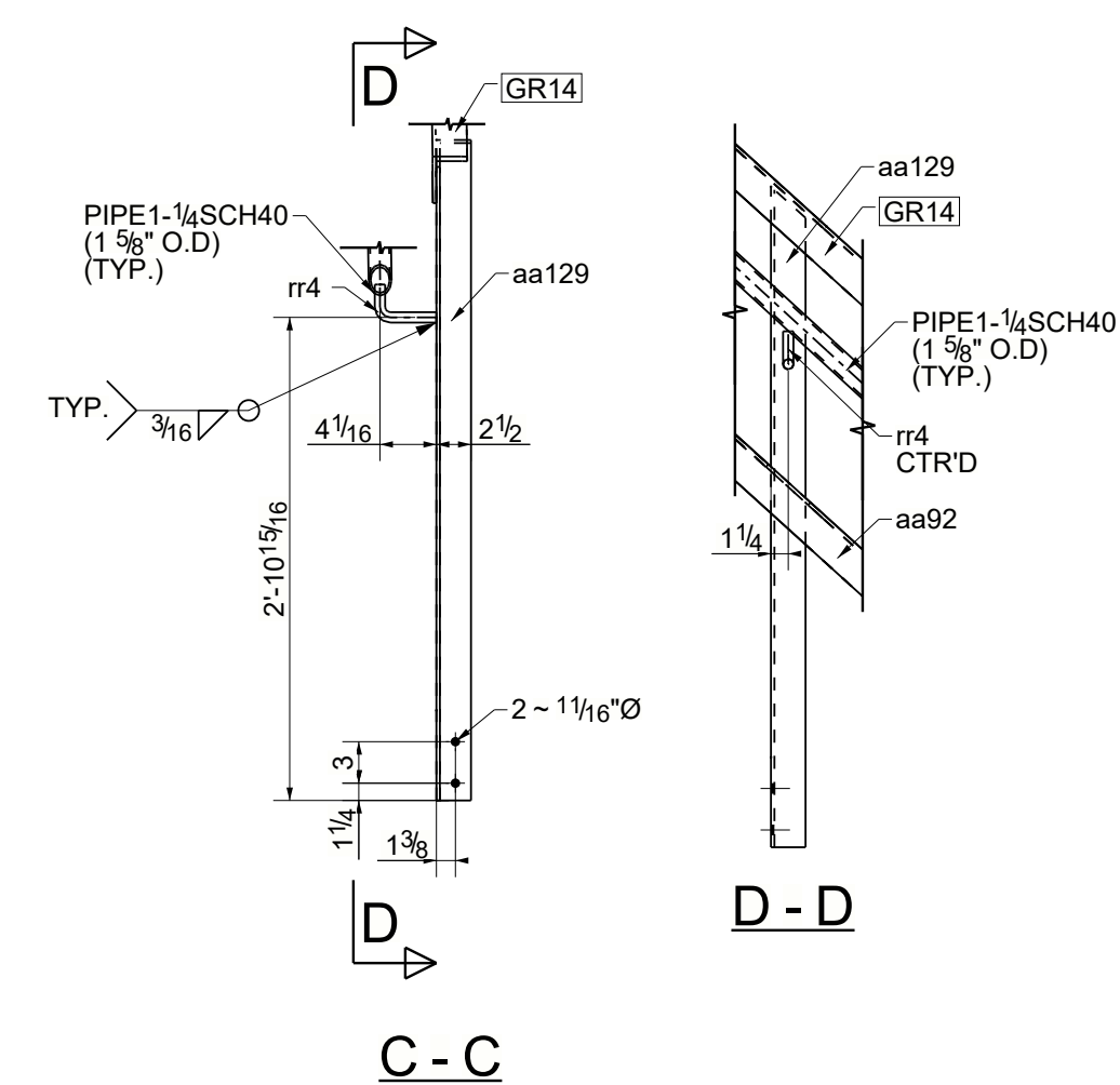
C - C
