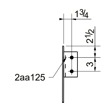
F - F
