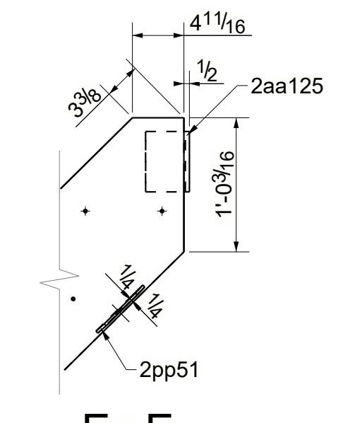
E - E
