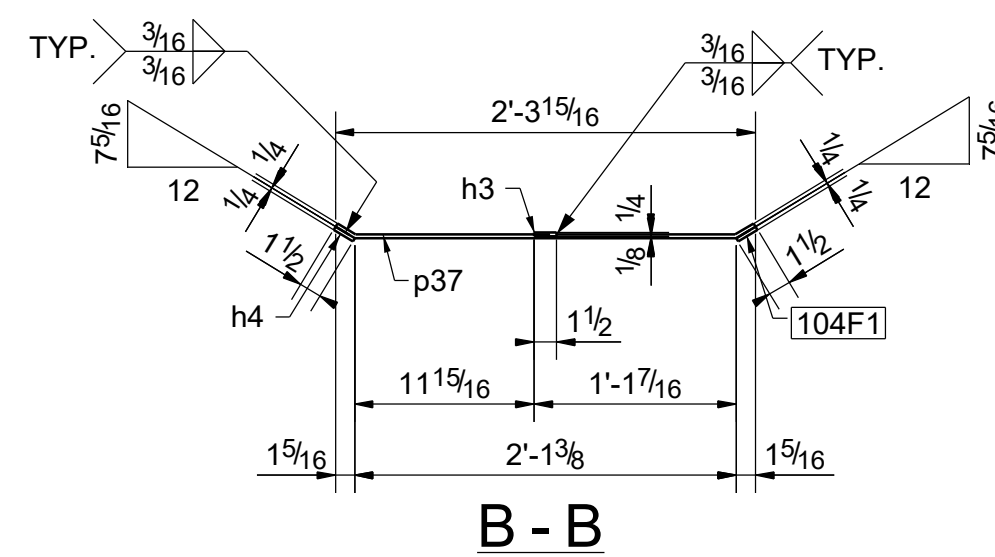
3 - FRAMES - 104F1
