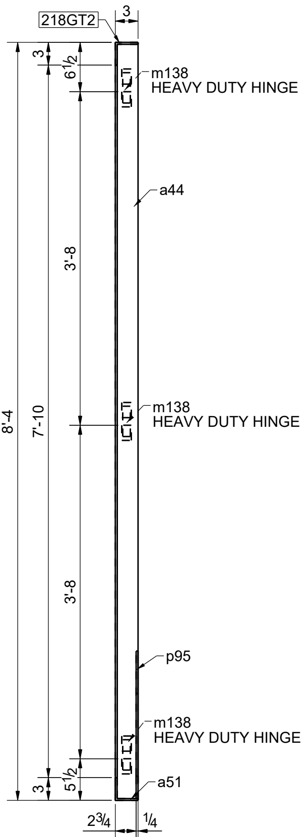
B - B
